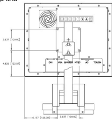
后视图
