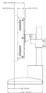
侧视图
