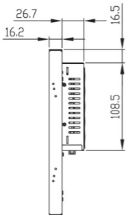
侧视图
