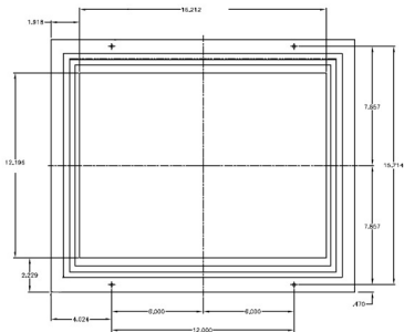
后视图
