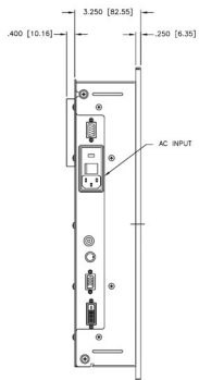
侧视图
