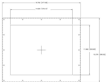
前视图
