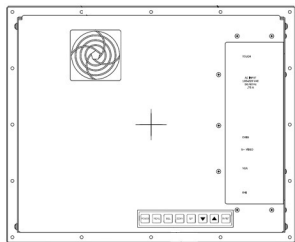
后视图
