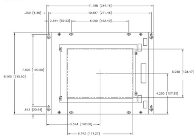
前视图
