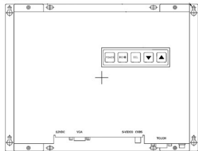
后视图
